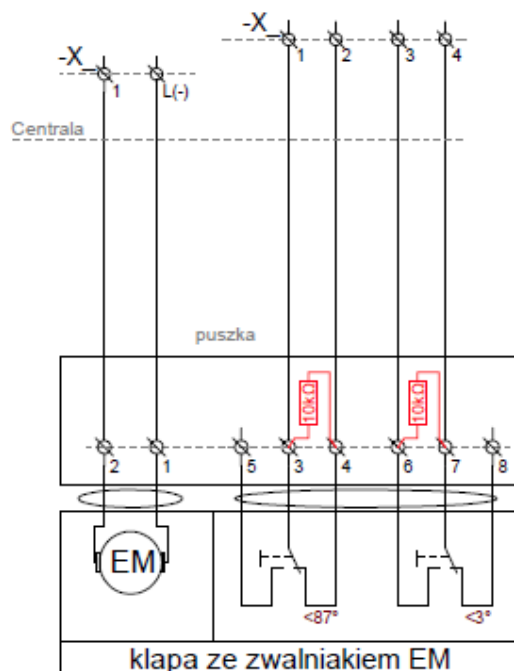
Rys. 22. Schemat siłownika ze zwalniającym.
