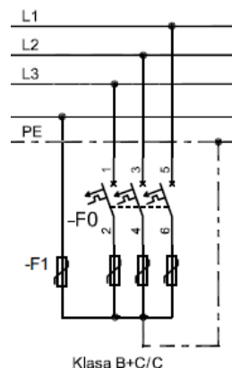
Rys. 5. Schemat zabezpieczenia przeciwprzepięciowego.
