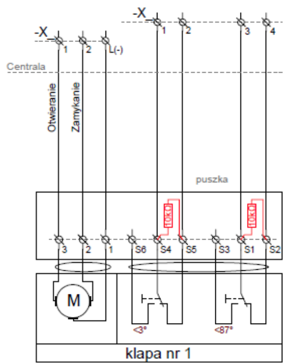
Rys. 17. Schemat siłownik z napędem elektrycznym, normalnie zamknięty.
